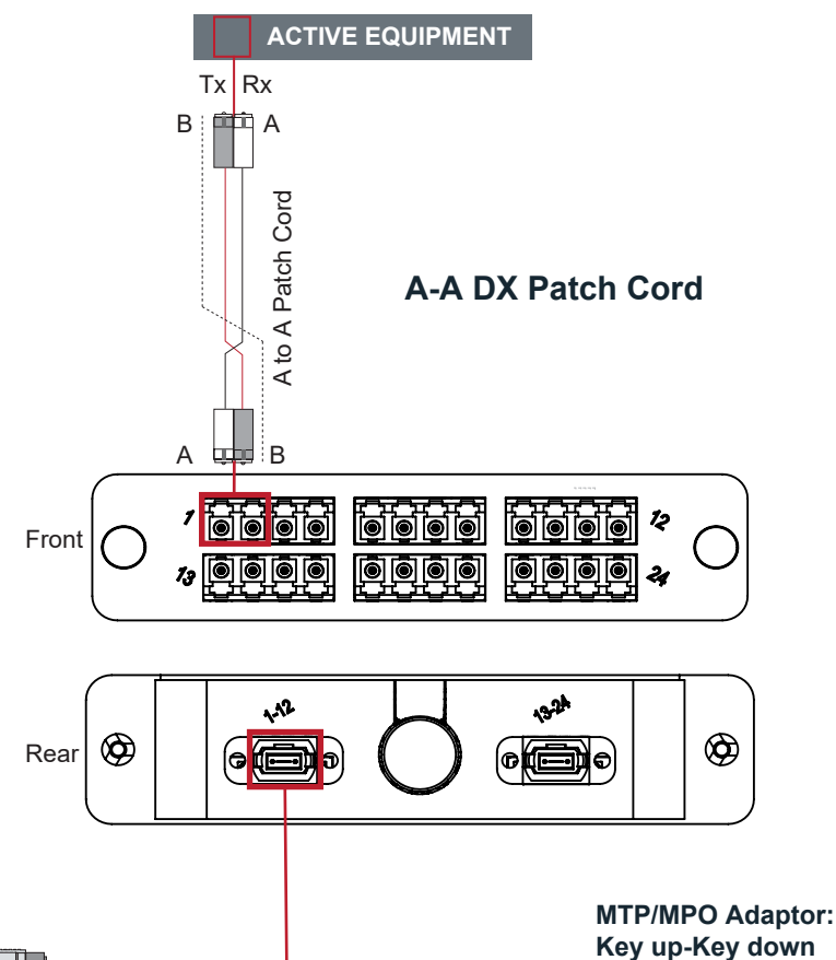
Type A MTP/MPO - LC Module
