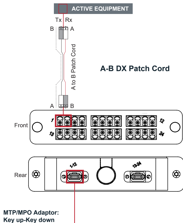
Type A MTP/MPO - LC Module
